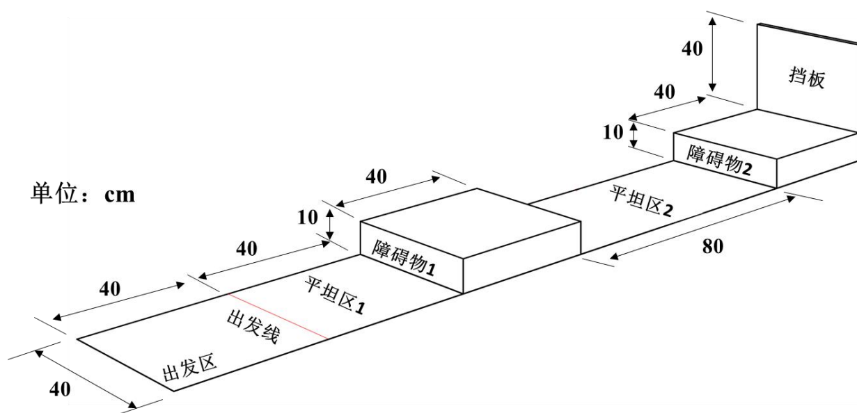
图 1 初赛赛道立体示意图
