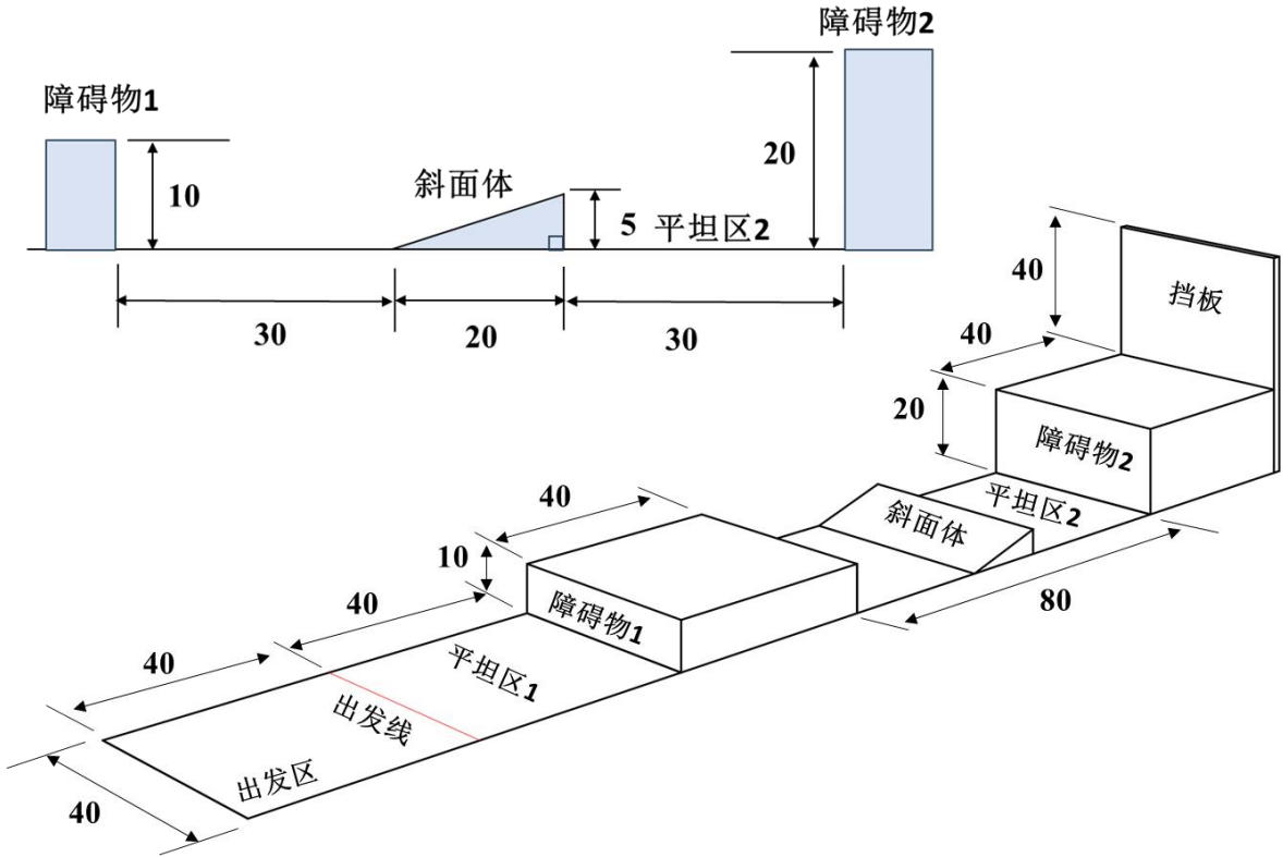
图 4 复赛赛道立体及局部示意图
